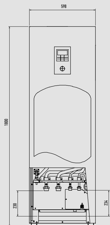
Frontansicht
