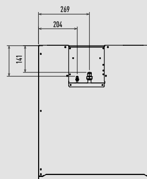
Draufsicht
