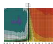
Mit Türluftschleier, aber zu hoher Luftstromgeschwindigkeit Dies führt zu Turbulenzen und Energieverlusten durch ineffektive Abschirmung der Türöffnung, die Kühlraumtemperatur wird zu hoch.
