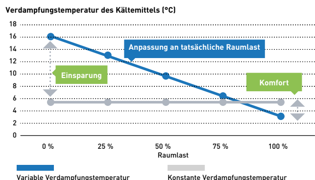
Lastabhängige, modulierende Regelung der Verdampfungstemperatur am Beispiel des Kühlbetriebs (für Heizbetrieb entsprechend)
