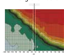
Ohne Türluftschleier Warme Luft dringt ungehindert in den Kühlraum ein, die Kühlraumtemperatur wird zu hoch.
