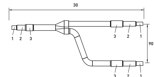
Flüssigkeitsleitung
