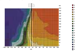
Mit Türluftschleier, aber falschem Ausblaswinkel Bei zu steilem Ausblaswinkel wird die warme Luft in den Kühlraum eingeblasen.
