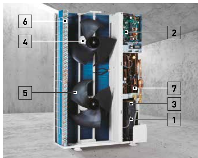
Dreilagig Leistungsstarker Wärmeübertrager Kompakter dreilagiger Wärmeübertrager: Trotz des um 15 % kleineren Gerätegehäuses bei den einphasigen 4-, 5- und 6-PS-Geräten ist die Oberfläche des neuen Wärmeübertragers genau so groß wie bei den Vorgängermodellen.
