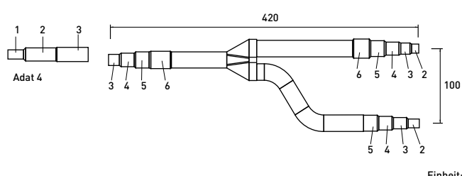
Flüssigkeitsleitung
