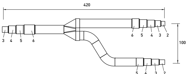
Gasleitung
