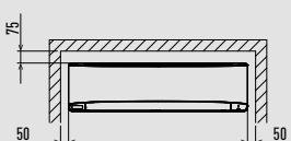
Mindestabstände für die Montage
