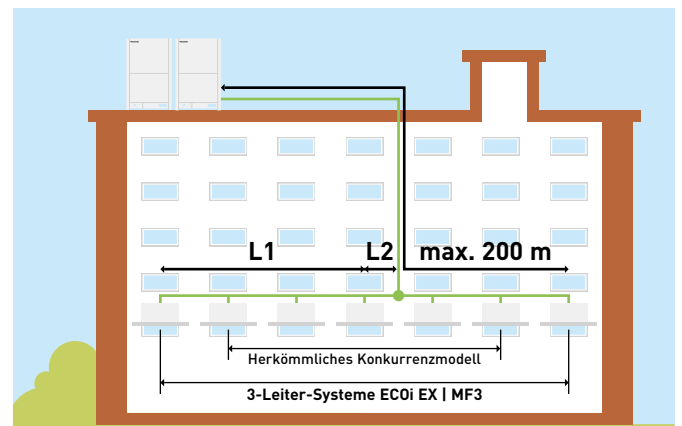
L1 = längster Rohrleitungsstrang, L2 = kürzester Rohrleitungsstrang, L1 - L2 = max. 40 m
